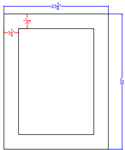
Door Size
